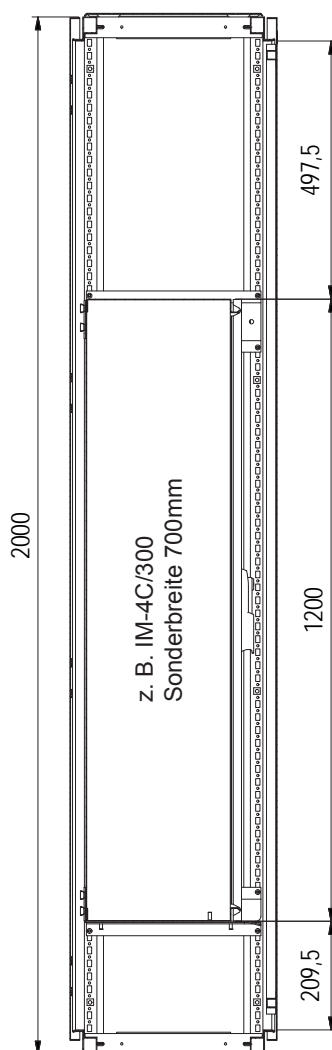
A-A (1 : 10)
