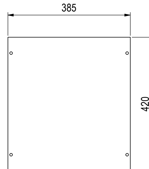
Montageplatte ( 1 : 7 )
