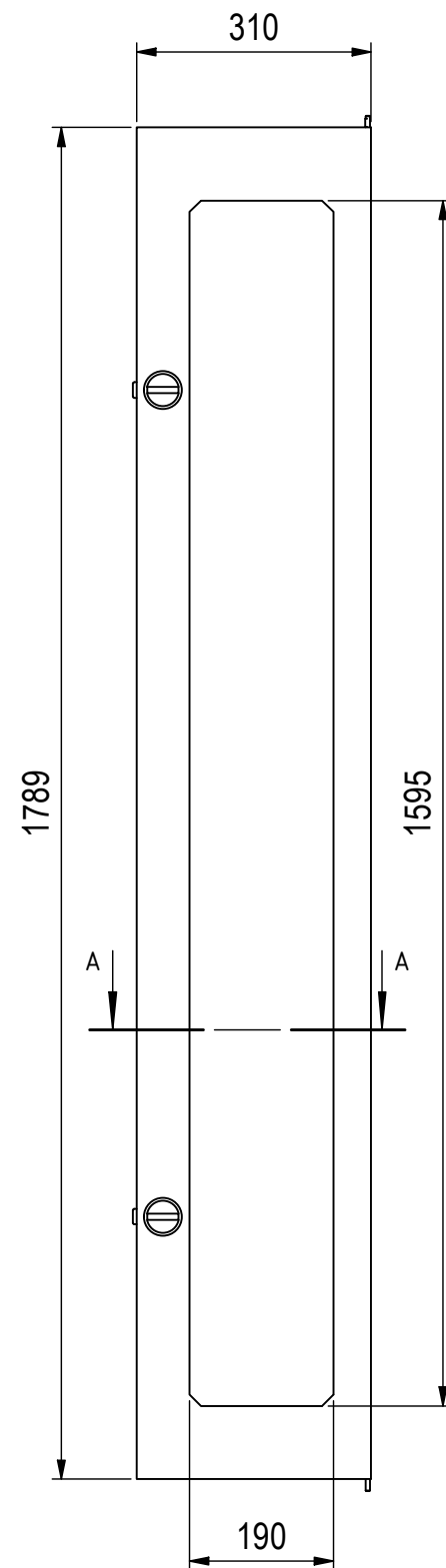
A-A ( 1 : 10 )
