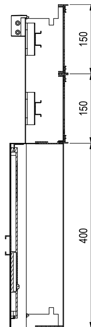
A-A ( 1 : 5 )
