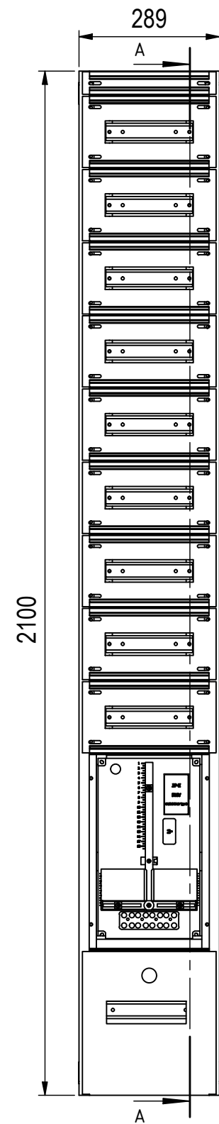
Hutschiene Vorzählerfach 214
