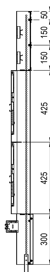
A-A ( 1 : 11 )
