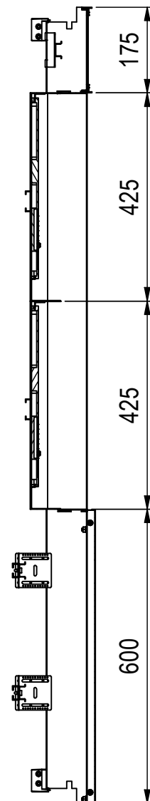
A-A ( 1 : 11 )
