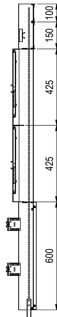
A-A ( 1 : 12 )
