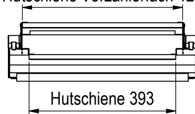
Hutschiene Vorzählerfach 429
