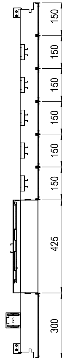
A-A ( 1 : 10 )
