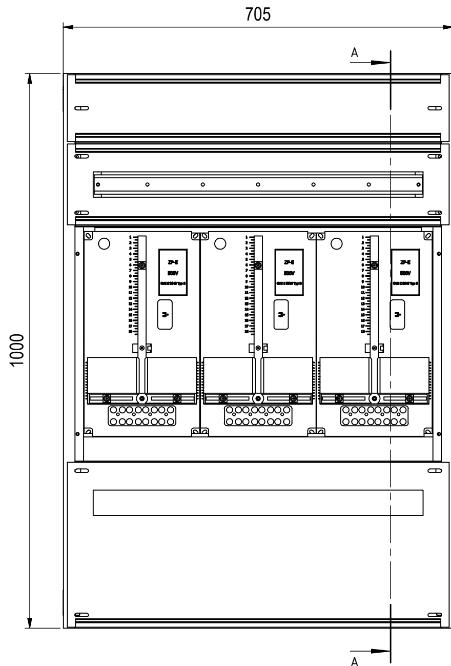
Hutschiene Vorzählerfach 629
