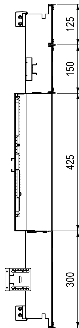
A-A ( 1 : 7 )
