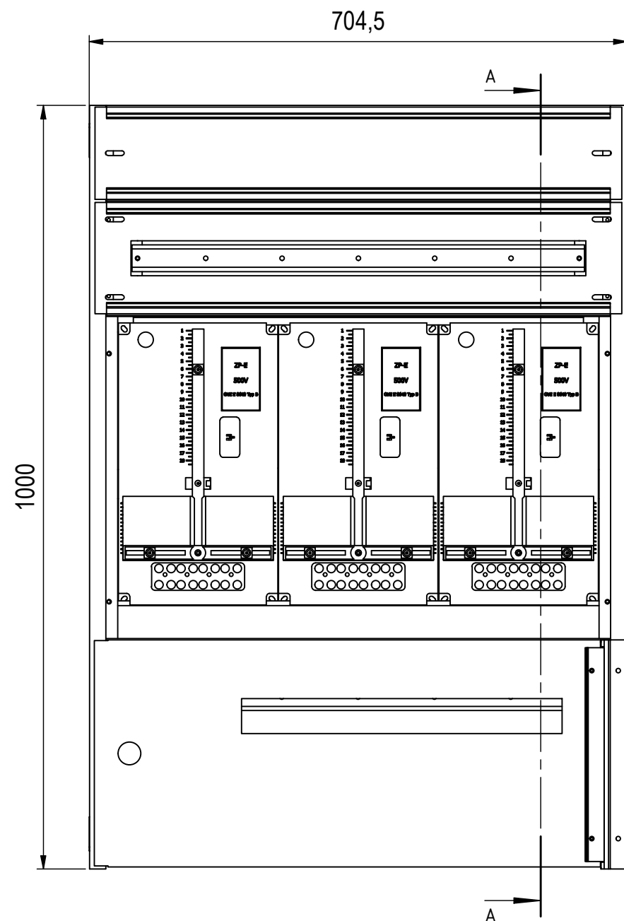
Hutschiene Vorzählerfach 629
