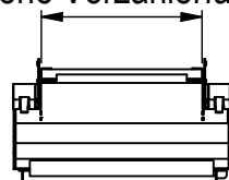
Hutschiene Vorzählerfach 214
