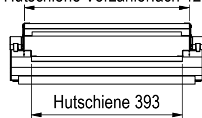
Hutschiene Vorzählerfach 429
