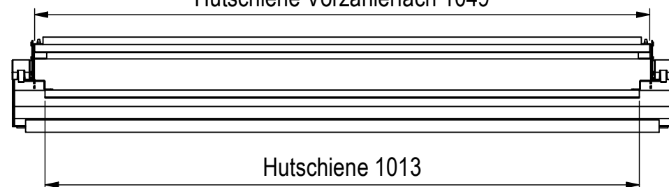
Hutschiene Vorzählerfach 1049
