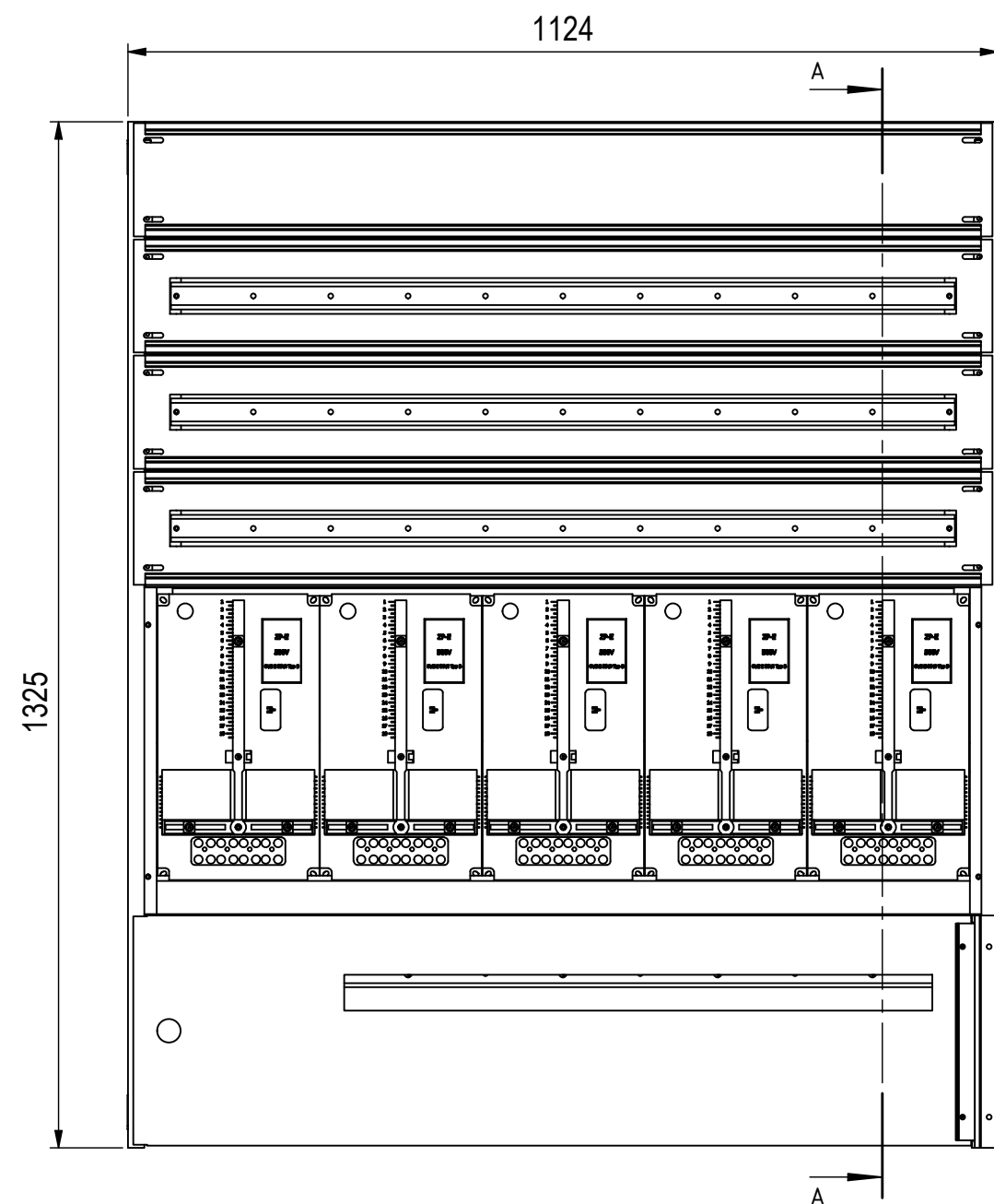
Hutschiene Vorzählerfach 1049
