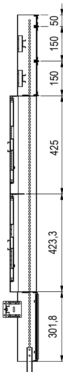
A-A ( 1 : 10 )
