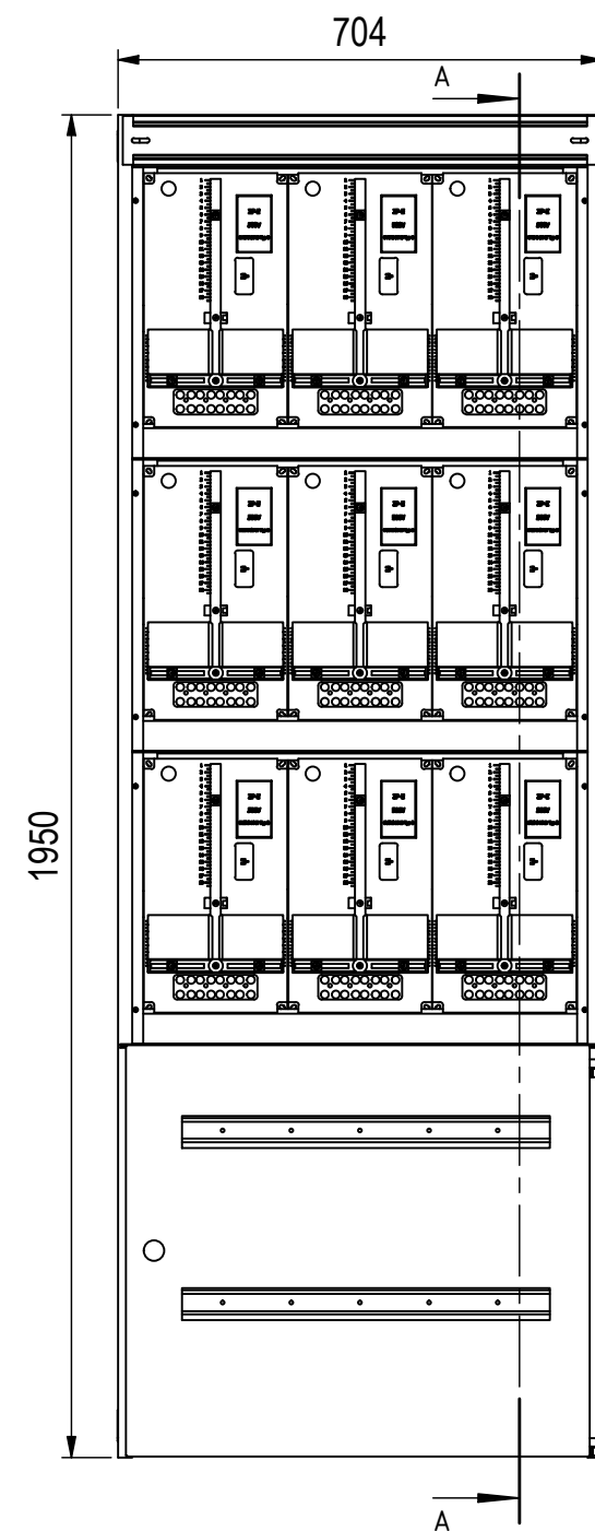
Hutschiene Vorzählerfach 629
