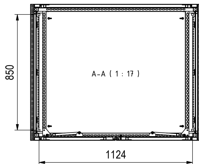
Bodenbefestigung □14mm
