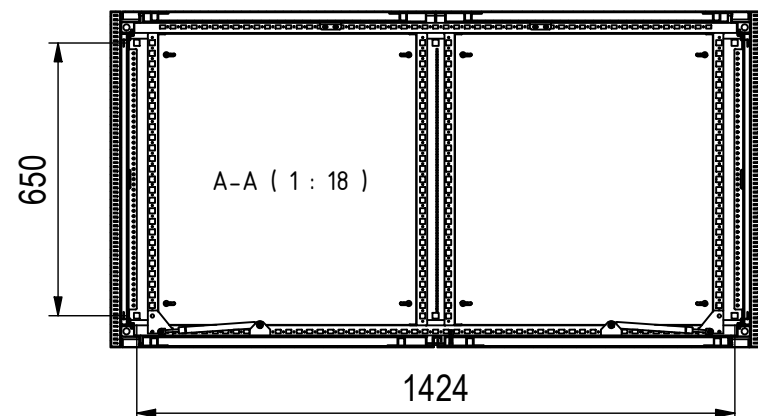
Bodenbefestigung □14mm
