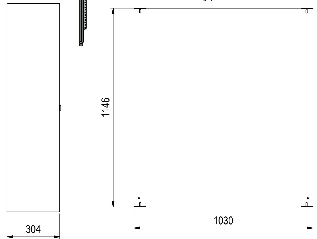
Montageplatte ( 1 : 13 )
