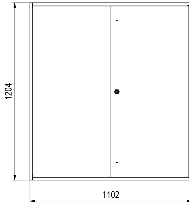
Innenschrank ( 1 : 13 )
