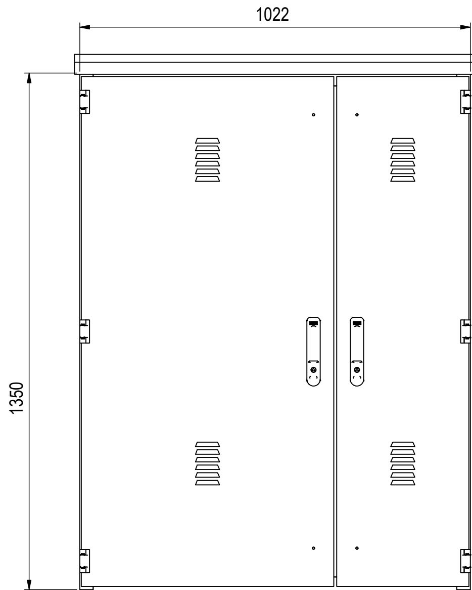
Innenschrank ( 1 : 10 )
