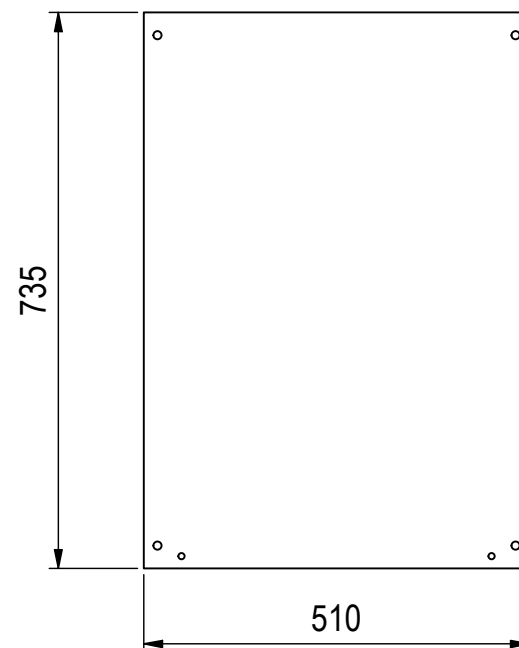
Montageplatte ( 1 : 10 )
