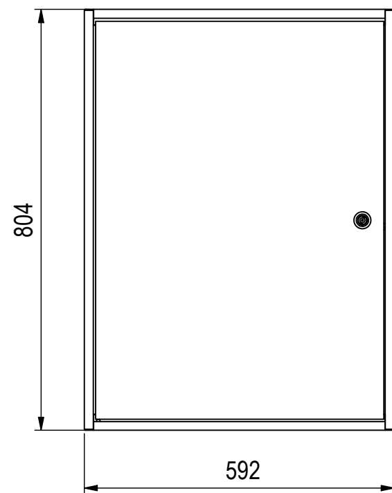
Innenschrank ( 1 : 10 )
