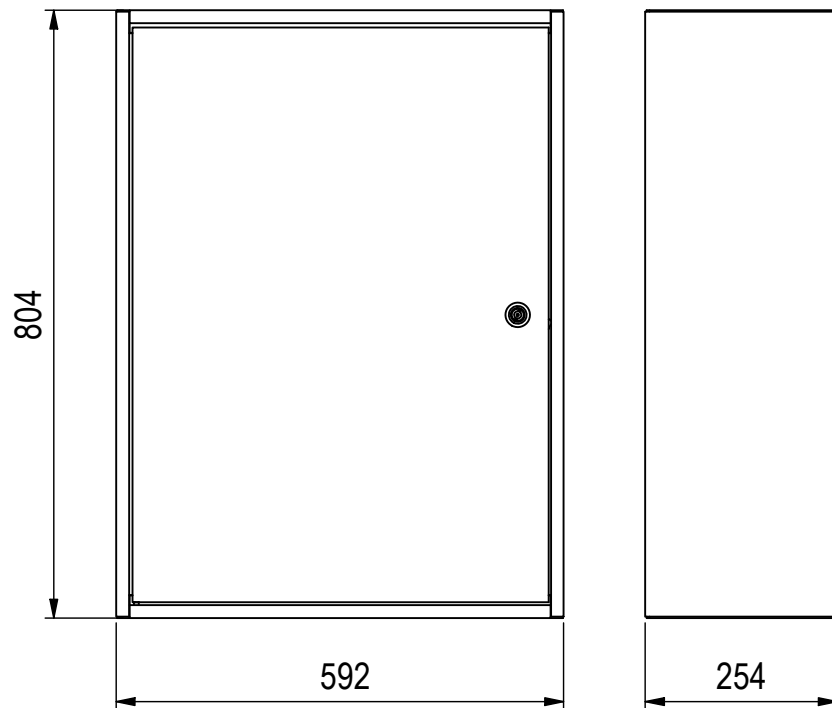
Innenschrank ( 1 : 10 )
