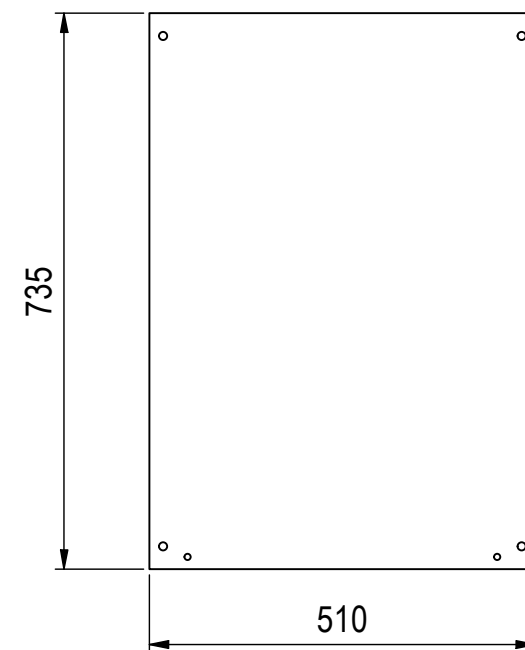
Montageplatte ( 1 : 10 )
