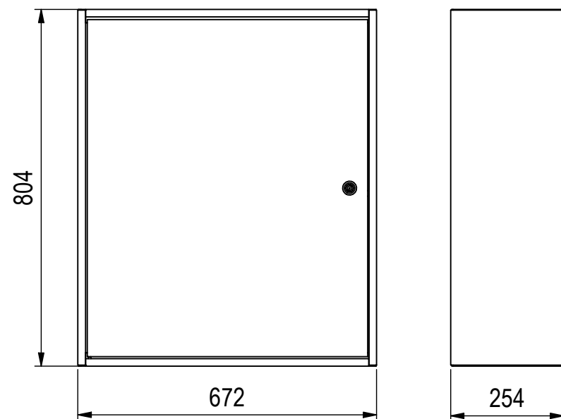
Innenschrank ( 1 : 12 )
