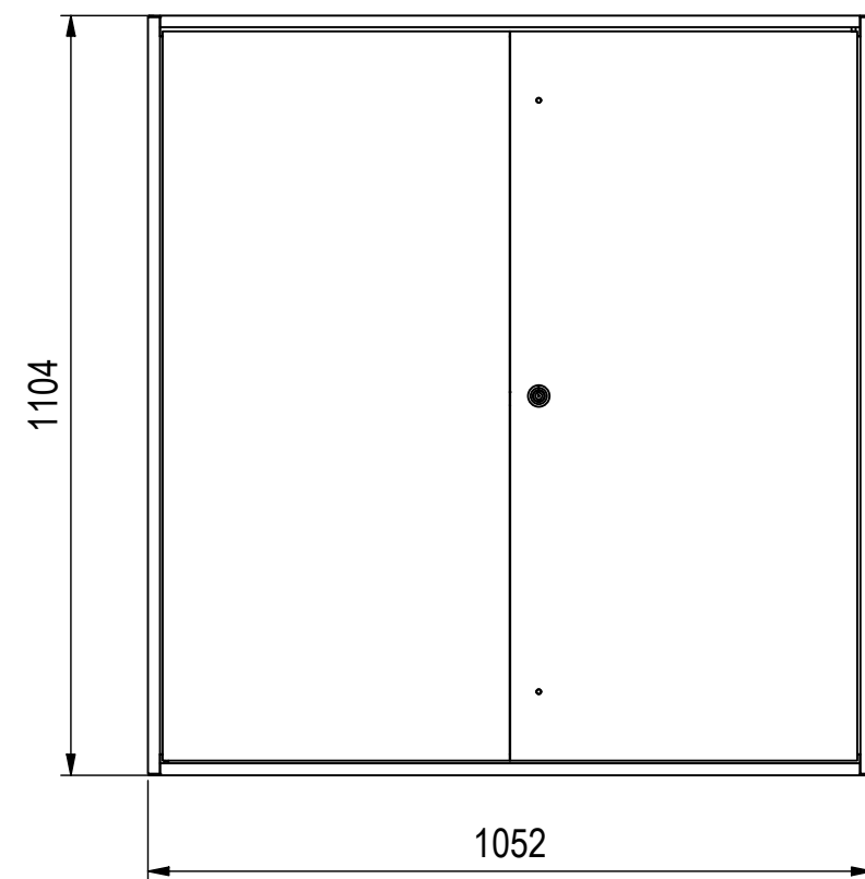
Innenschrank ( 1 : 12 )
