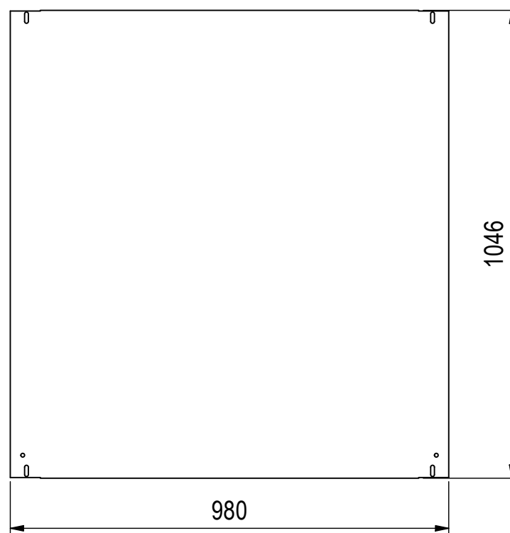
Montageplatte ( 1 : 12 )
