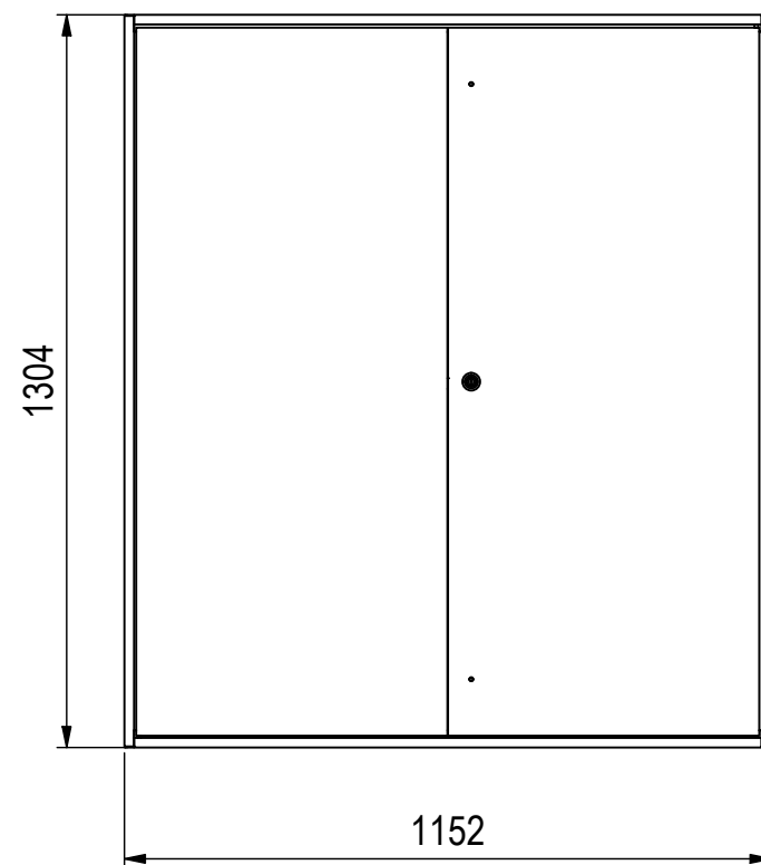
Innenschrank ( 1 : 15 )
