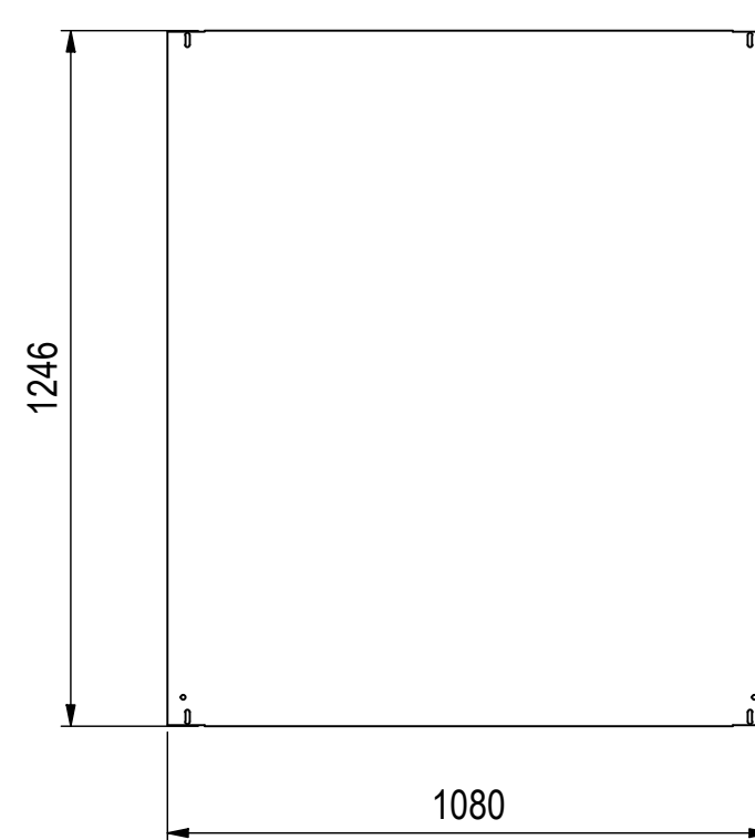
Montageplatte ( 1 : 15 )
