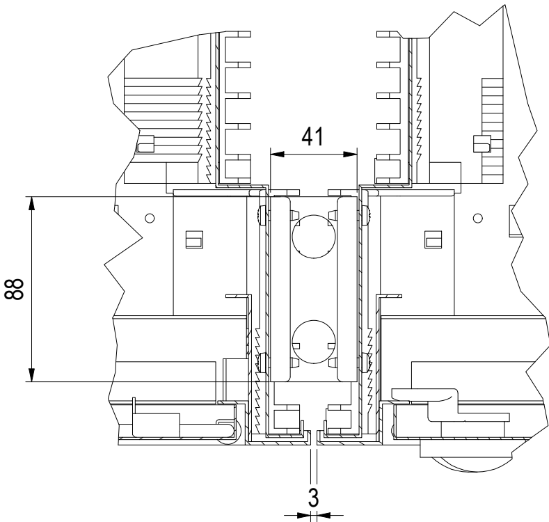
E ( 0,40 : 1 )
