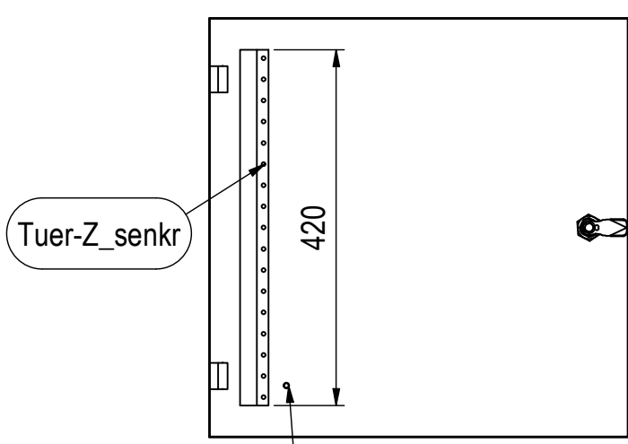
ANSICHT TÜR
