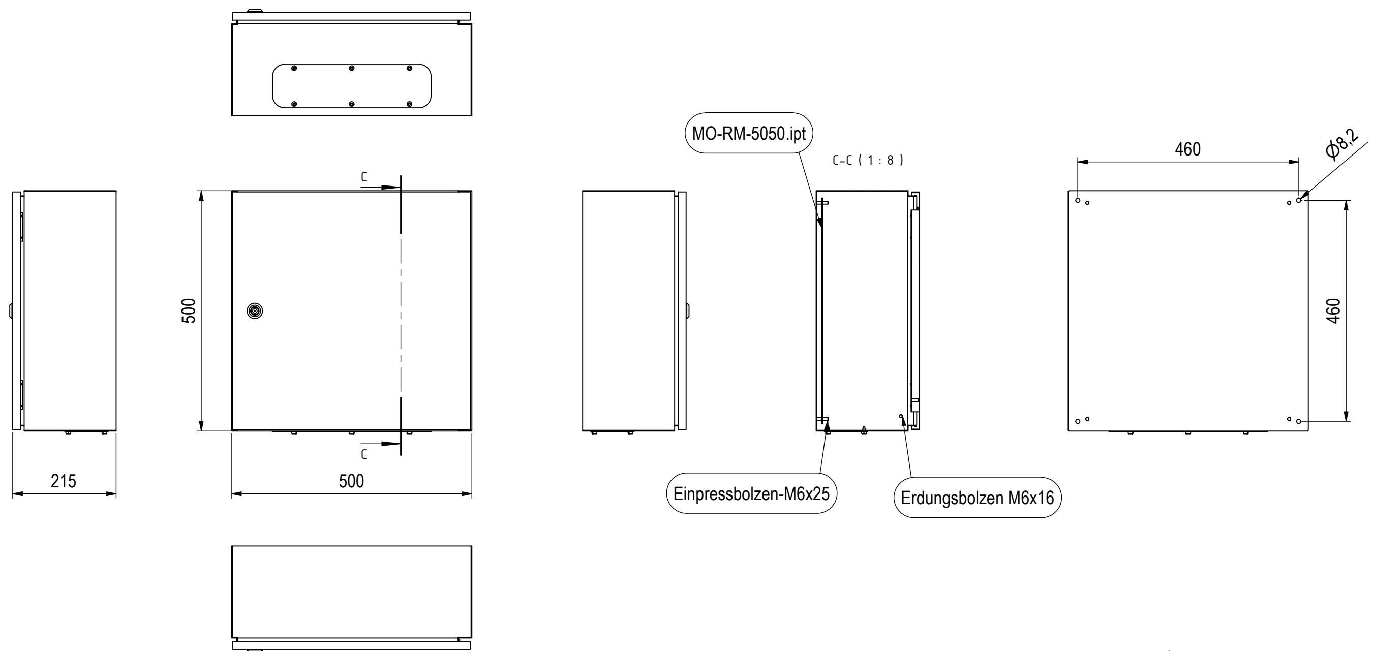
ANSICHT TÜR
