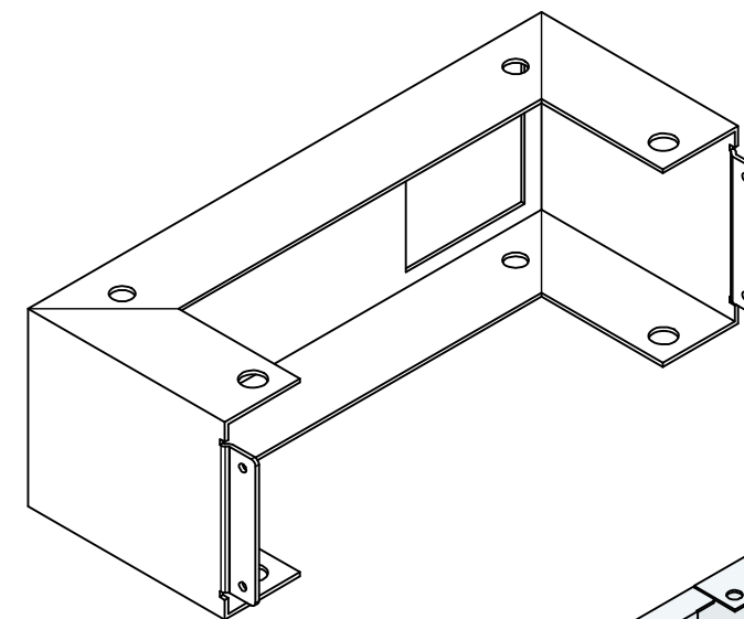
SO-Blende_AMST-D100
