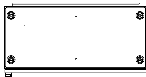
Bodenbefestigung □14mm
