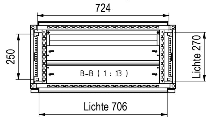
Bodenbefestigung □14mm
