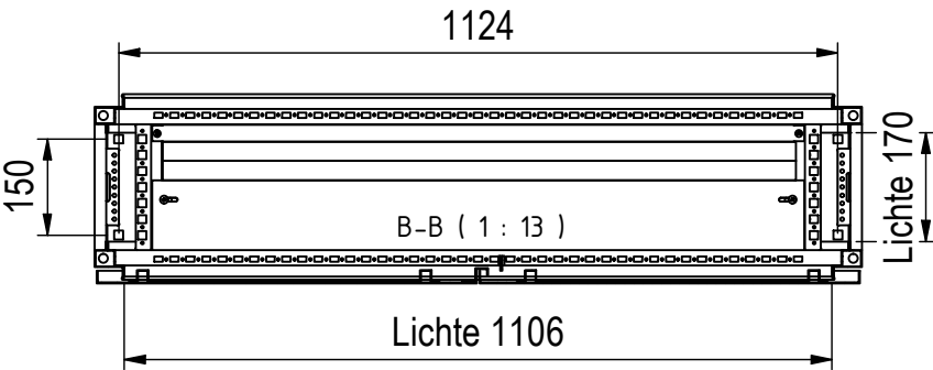
Bodenbefestigung □14mm
